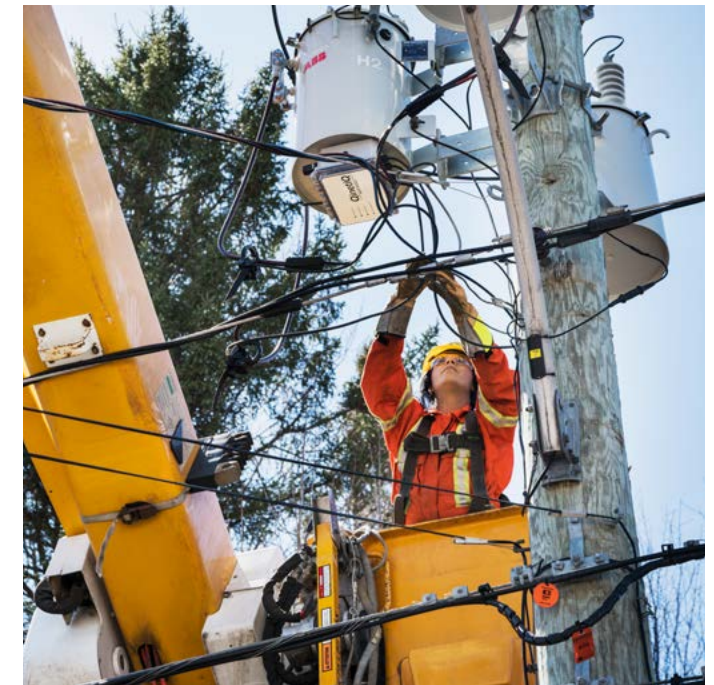
Installation du système MILE (maintenance intelligente de lignes électriques) sur une ligne de distribution dans les Laurentides.
