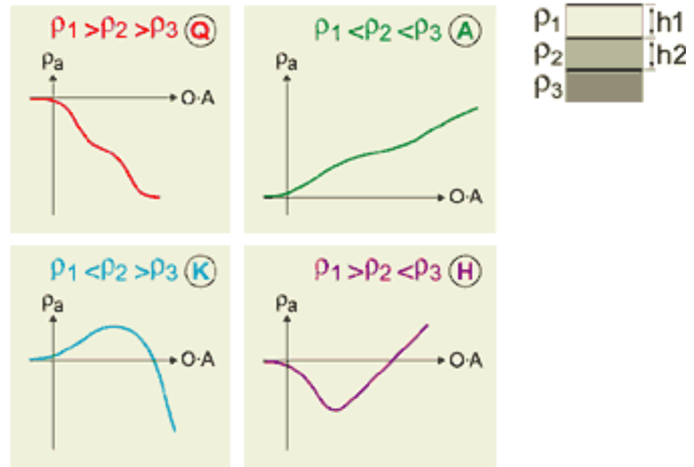
Courbes types pour un modèle à 3 couches
