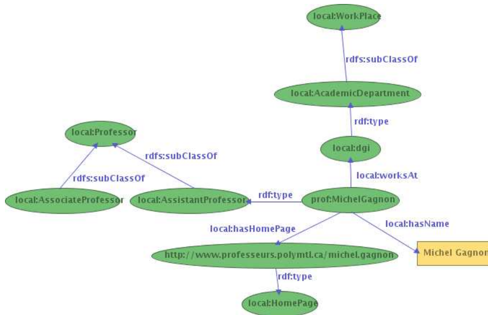
FIGURE 8 – Hiérarchie de classes
