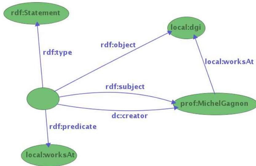
FIGURE 6 – Exemple de réification
