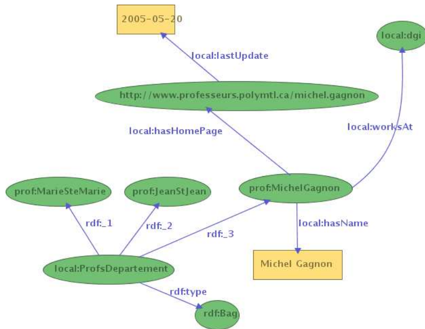
FIGURE 5 – Exemple de description de conteneur
