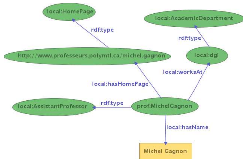
FIGURE 4 – Exemple de graphe RDF avec types de ressources identifiés
