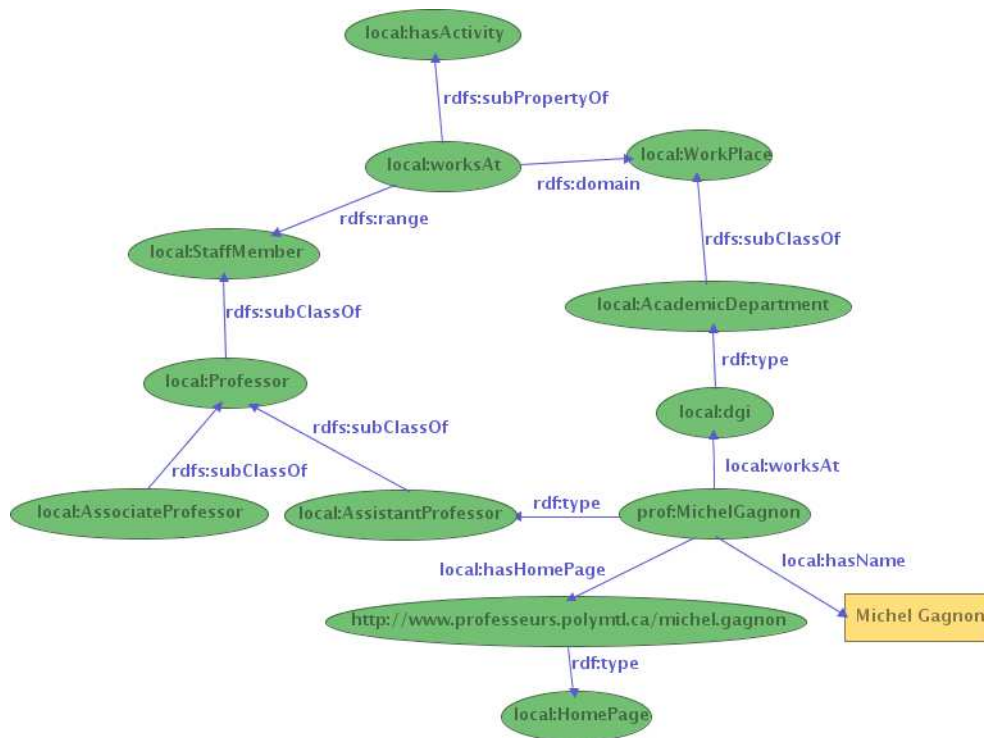
FIGURE 9 – Hiérarchie de propriétés
