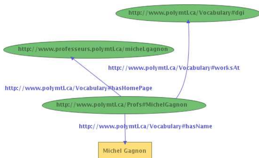
FIGURE 2 – Un premier exemple
