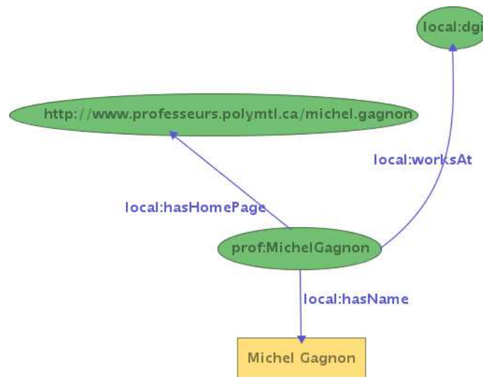
FIGURE 3 – Exemple avec utilisation de préfixe
